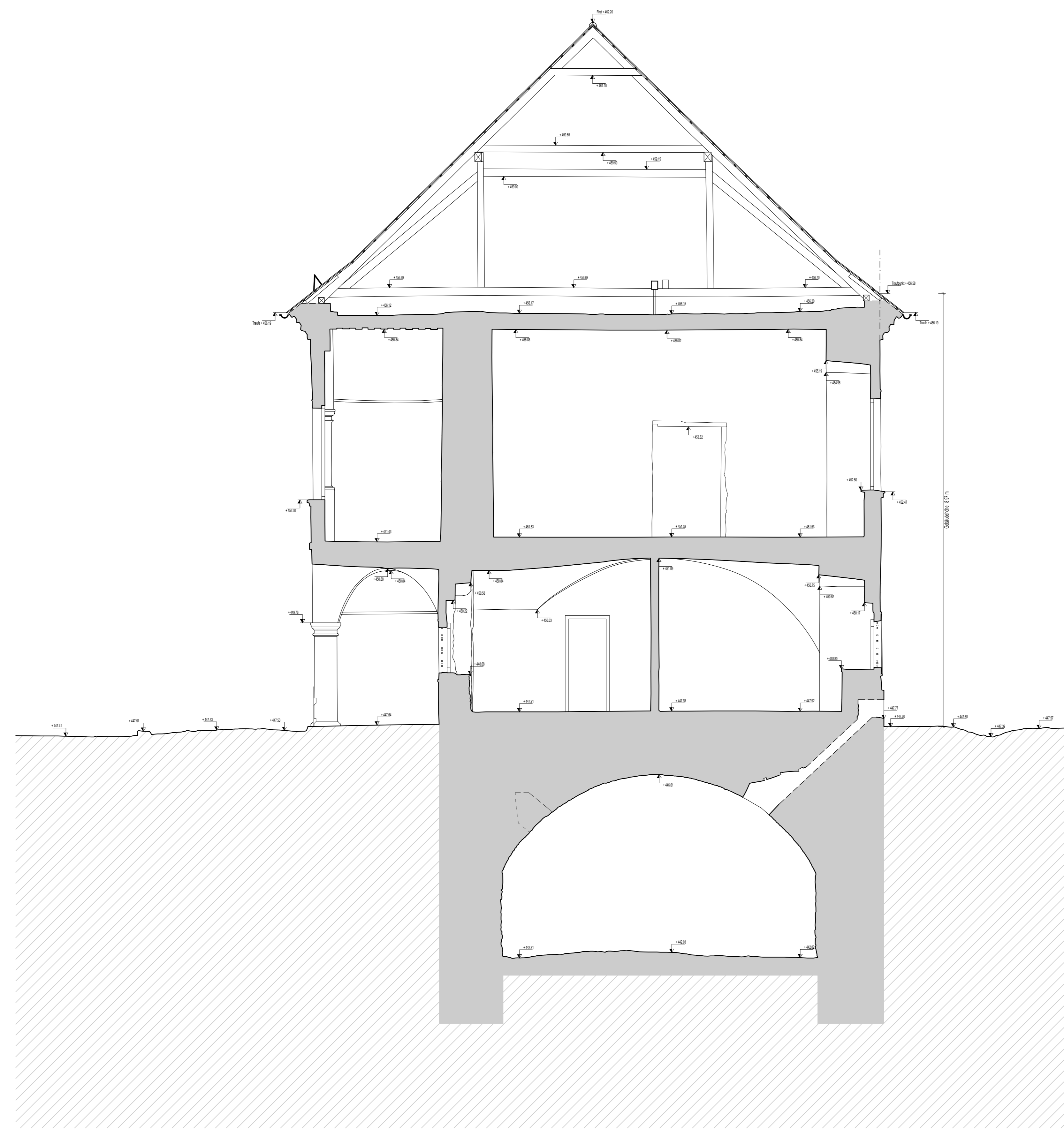
Querschnitt C-C
