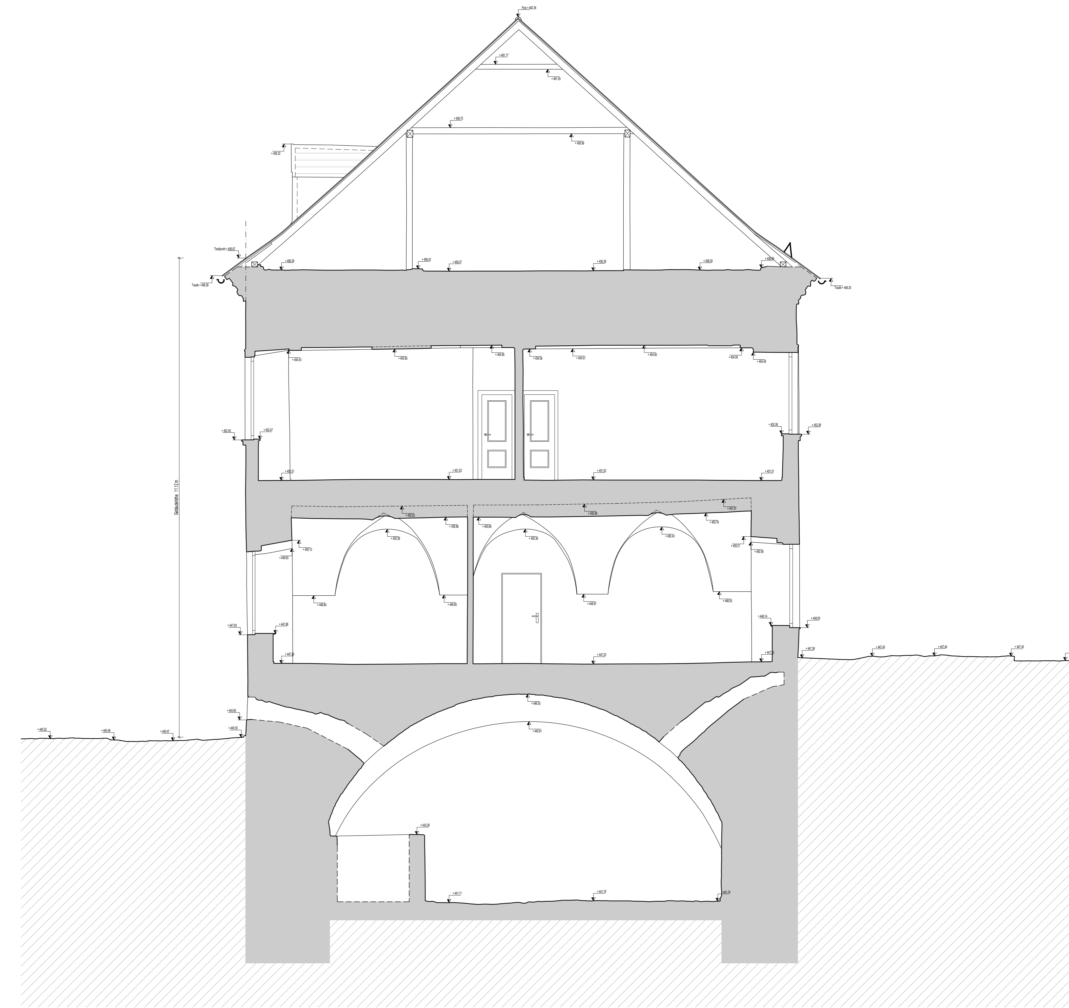
Querschnitt D-D
