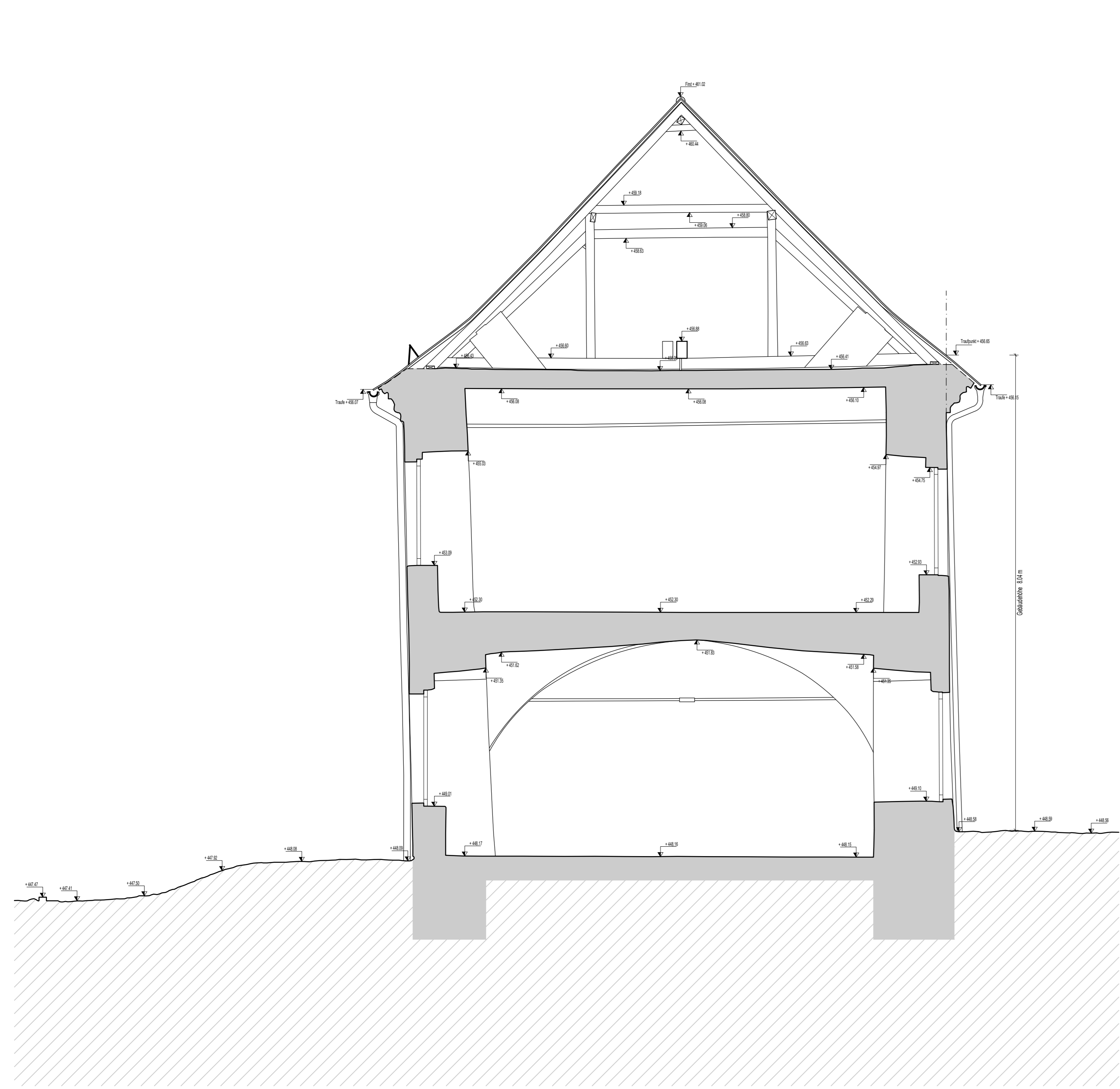
Querschnitt B-B
